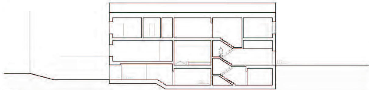
Querschnitt B-B
